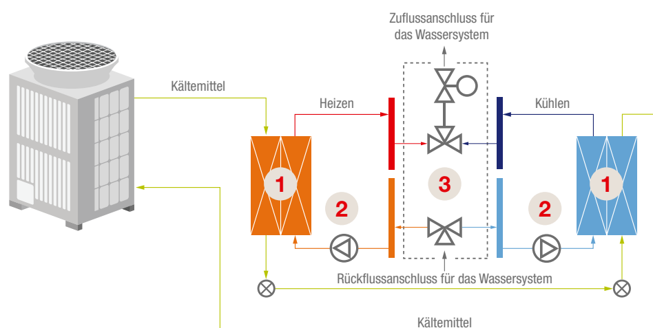
Hybrid BC-Übersicht
